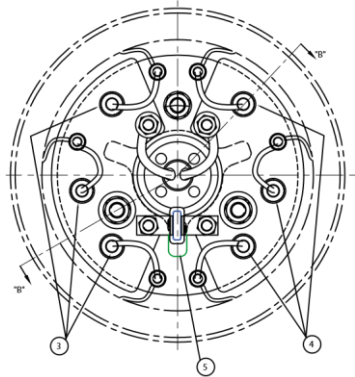
ROTATING RECTIFIER ASSEMBLY
