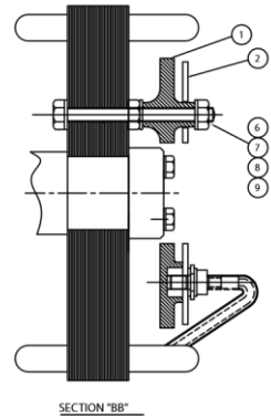
ROTATING RECTIFIER ASSEMBLY
